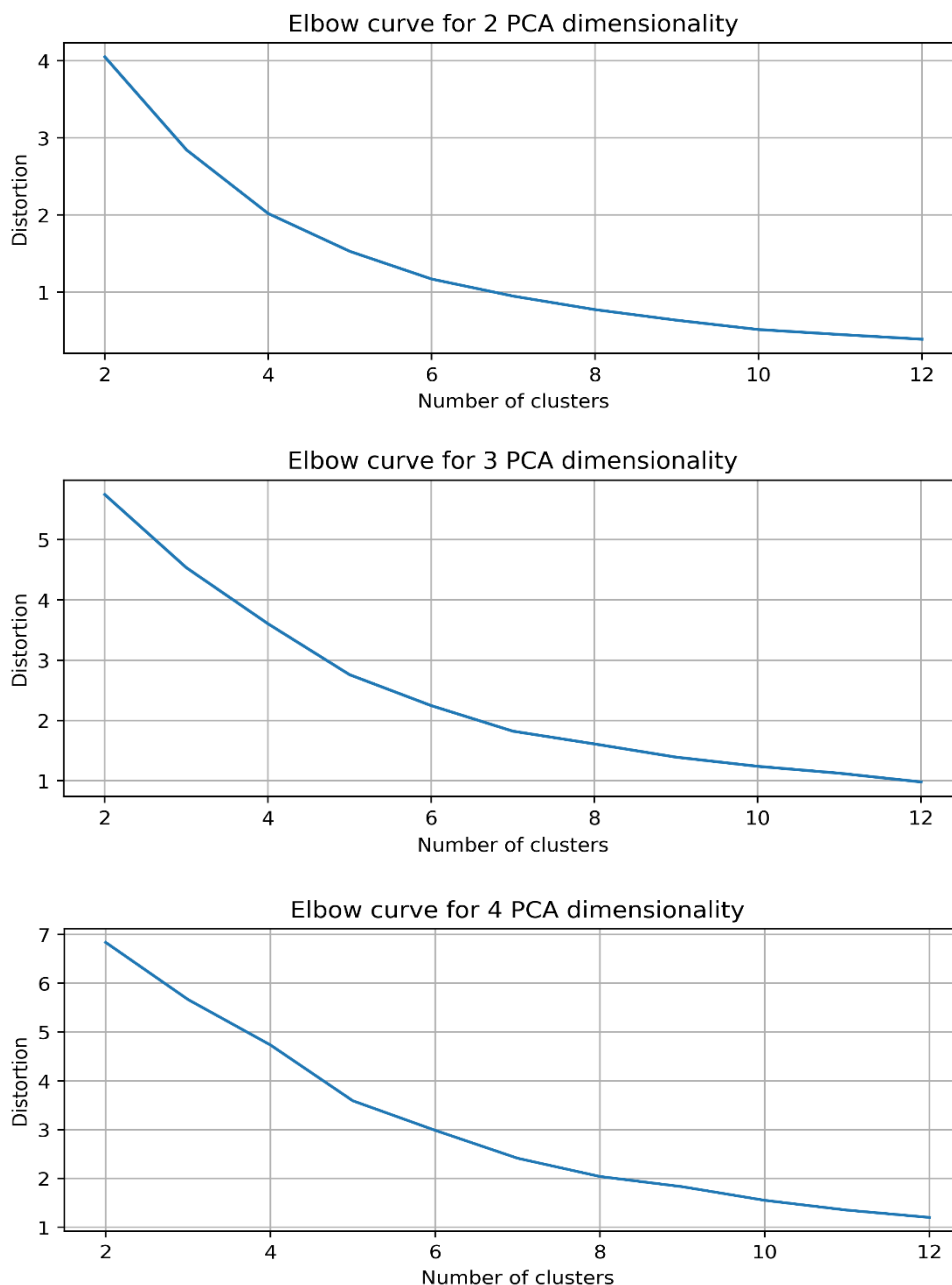
Εικόνα 40: Elbow curve for different PCA components
