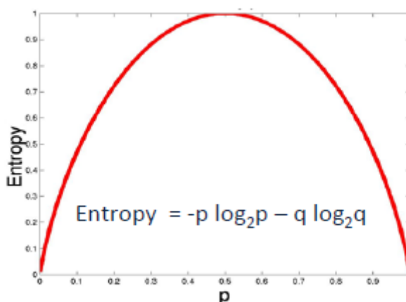
Εικόνα 5: Entropy
