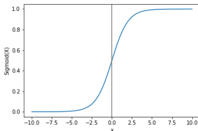
Εικόνα 2: Σιγμοειδής συνάρτηση
